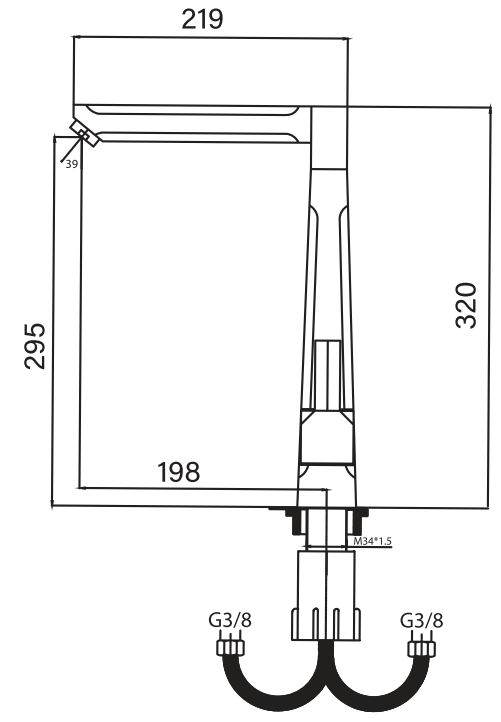
Sink faucet ظرفشویی
